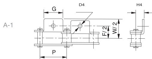
Aleta 90° 2 taladros 1 lado
