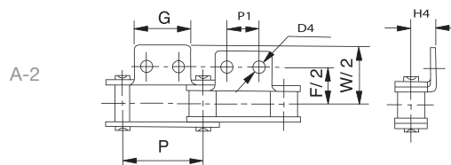
Aleta 90° 2 taladros 1 lado
