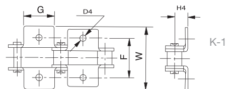
Aleta 90° 1 taladro 2 lados
