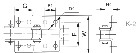
Aleta 90° 2 taladros 2 lados
