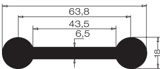
Perfil H - Negro H Profile - Black Profil H - Noir
