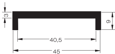
Perfil U-45 - Negro U-45 Profile - Black Profil U-45 - Noir
