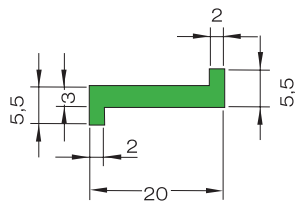
Perfil Z - Verde Z Profile - Green Profil Z - Vert
