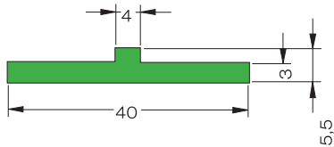
Perfil T - Verde T Profile - Green Profil T - Vert
