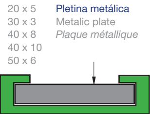
Perfil Z - Verde Z Profile - Green Profil Z - Vert
